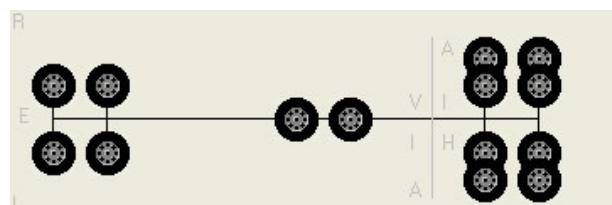
Standard 4-Achs Baustellenfahrzeug mit 2 Reserverädern
